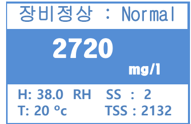
< 3단계 Main화면 >
