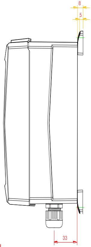
< Figure 9-0-2. 측면부 구성 >
