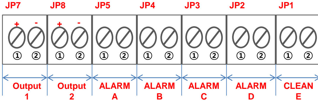
< Figure 10-3. 알람 & 세정기 Relay 연결 단자 구성 >
