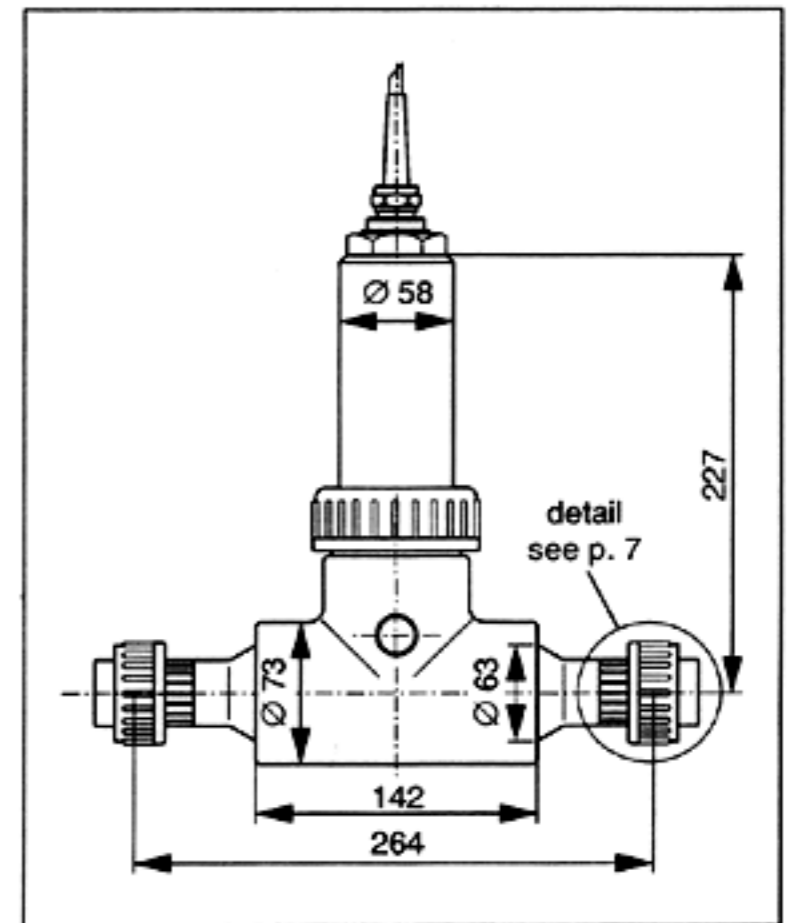
Dimensions OUA 250-A/-B
