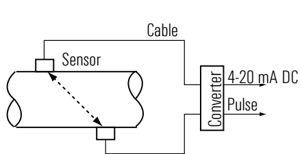
1-path system (Z method)
